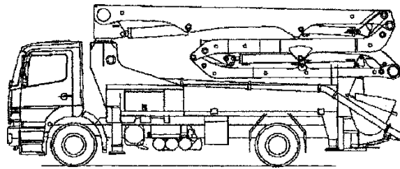
Esempio di pompa per calcestruzzo
