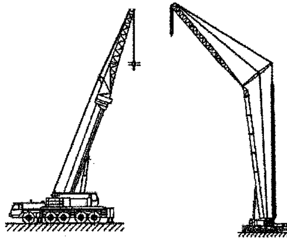
Esempi di gru mobili su ruote con falcone telescopico o brandeggiante
